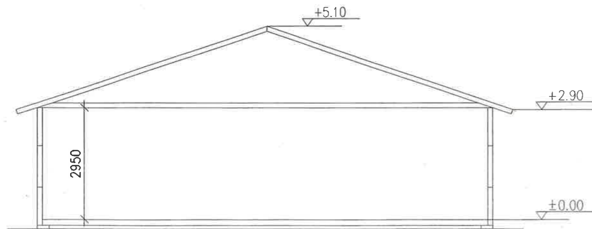
LEIKKAUS A - A
